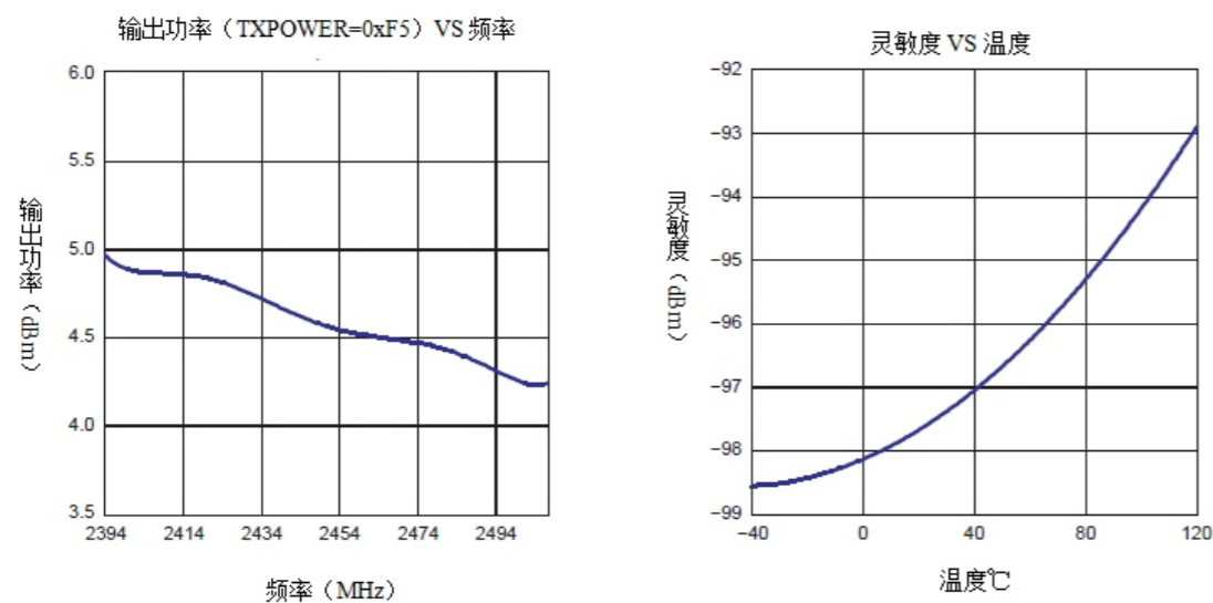
图1 输出功率 (TXPOWER=0xF5) VS频率曲线图
